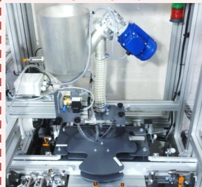
OPTION MLP328 - DOSAGE DE PRODUIT A FORTE VISCOSITE
